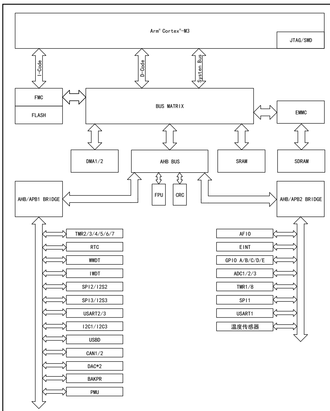
图 2 APM32E103VET6S 系统框图
